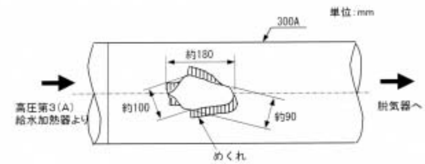
損傷部寸法
