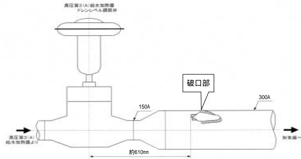
損傷部位置図
